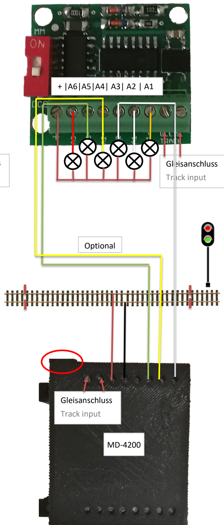
Mit MFB-Modul (MD-4200)
