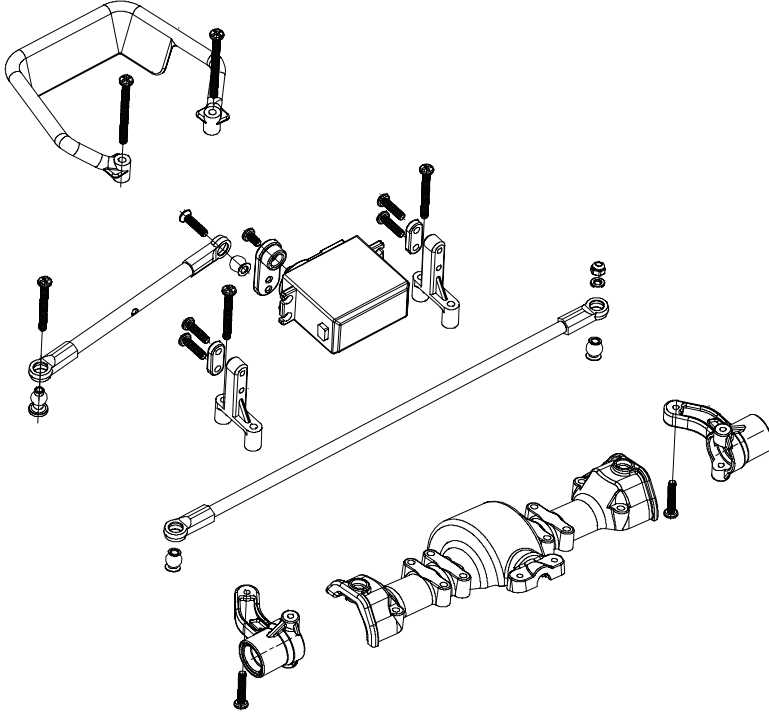
500502046 Servo f. 4WD Lenkung inkl. V-Kabel / Servo f. 4WD Steering incl. V-cable
